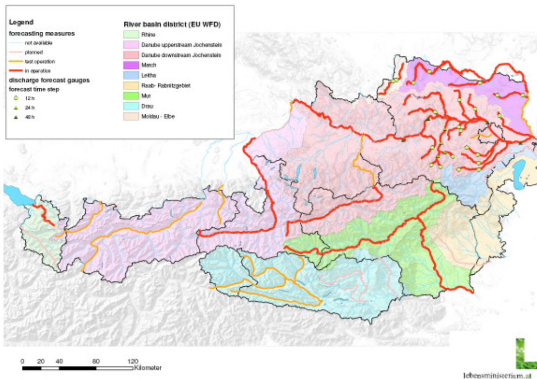
Abbildung 3: Hochwasservorhersagemodelle in Österreich und Prognoseergebnisse im Internet
